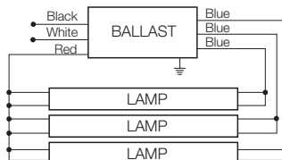
QUICKTRONIC 3x32
