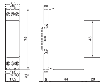
fig. 4. dimensions (mm)
