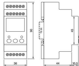
fig. 4. Dimensions (mm)
