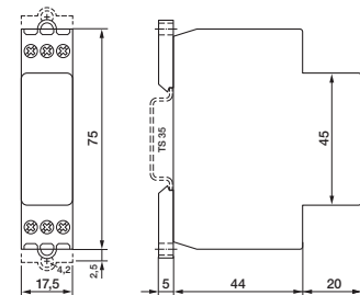
fig. 4. Dimensions (mm)
