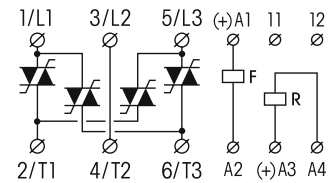
fig. 1. Wiring diagram
