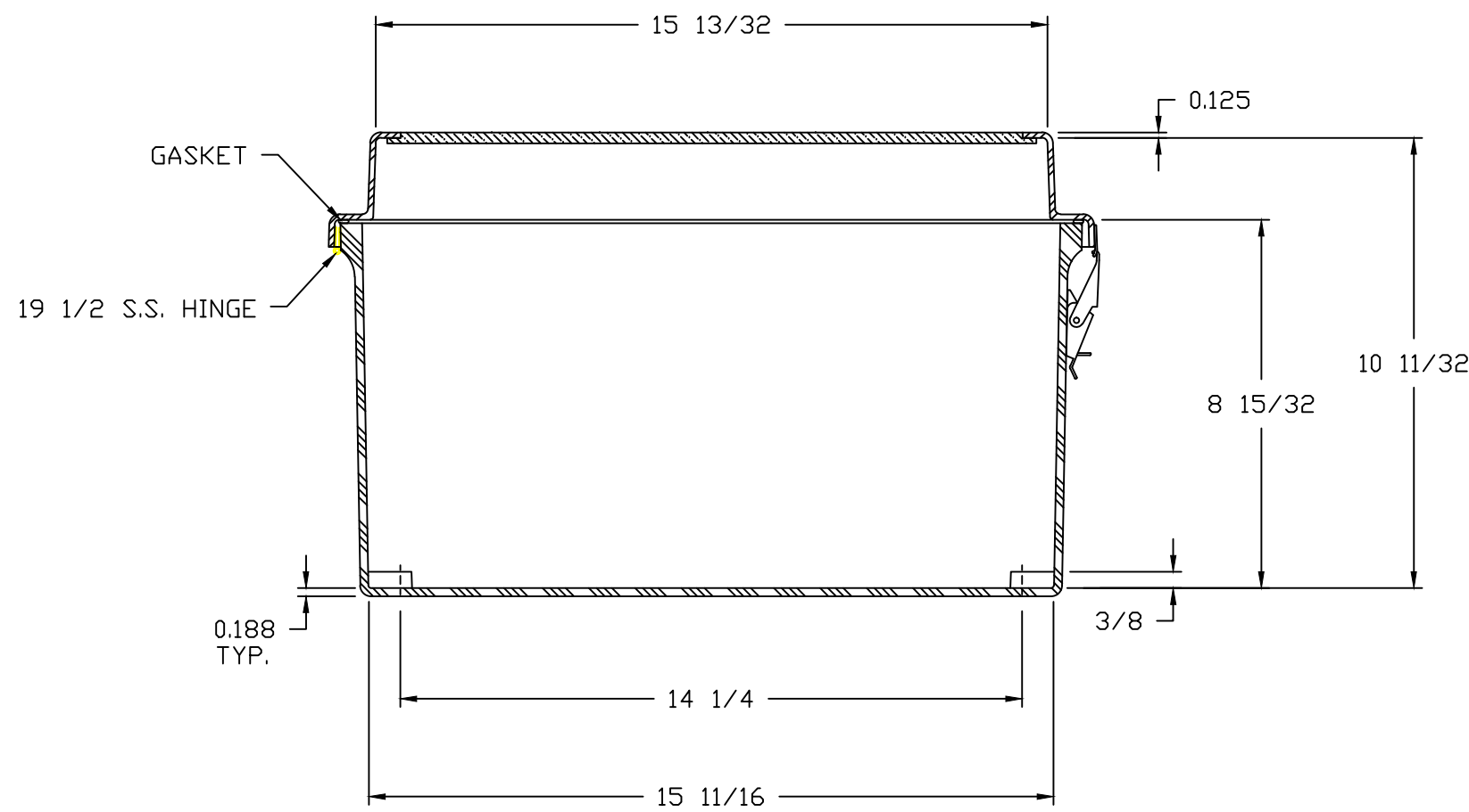
SECTION A-A
