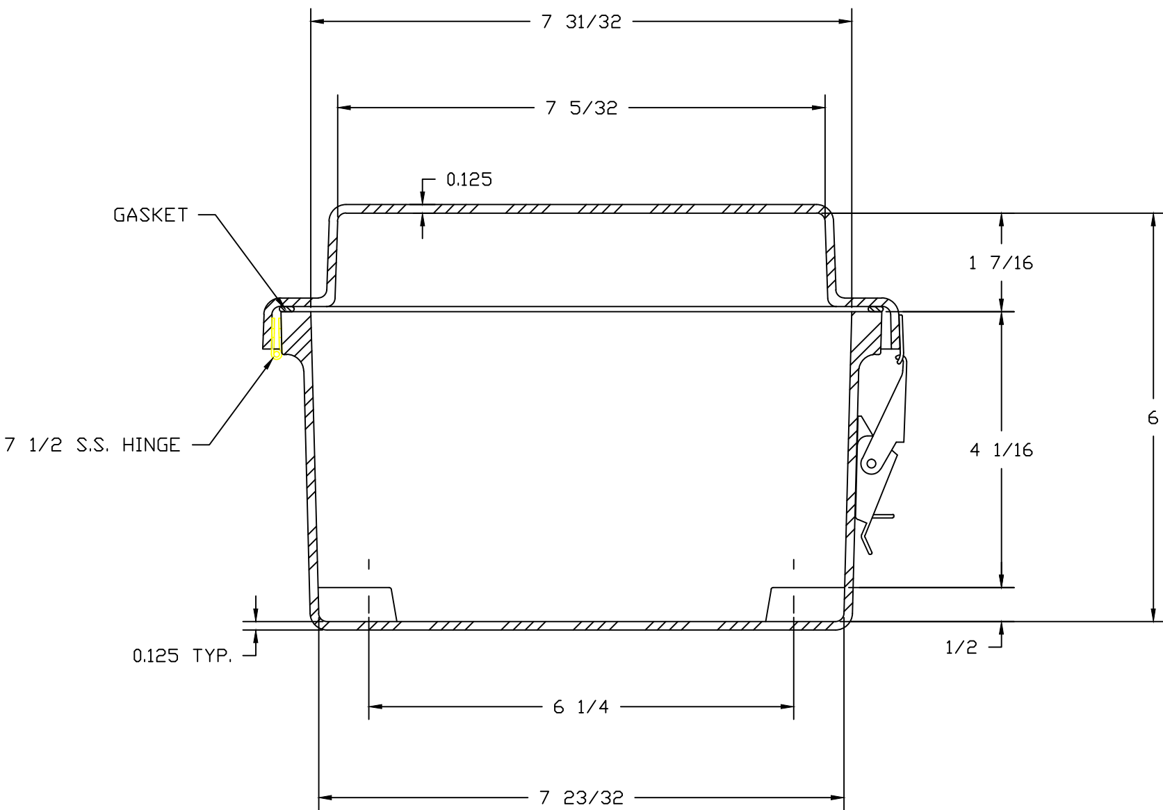
SECTION A-A
