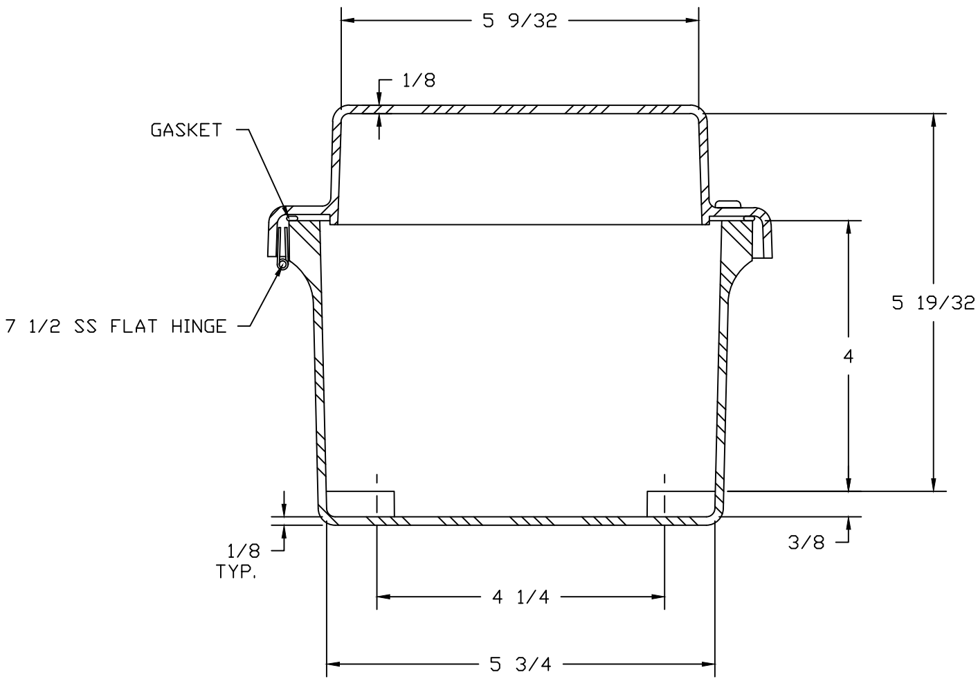
SECTION A-A
