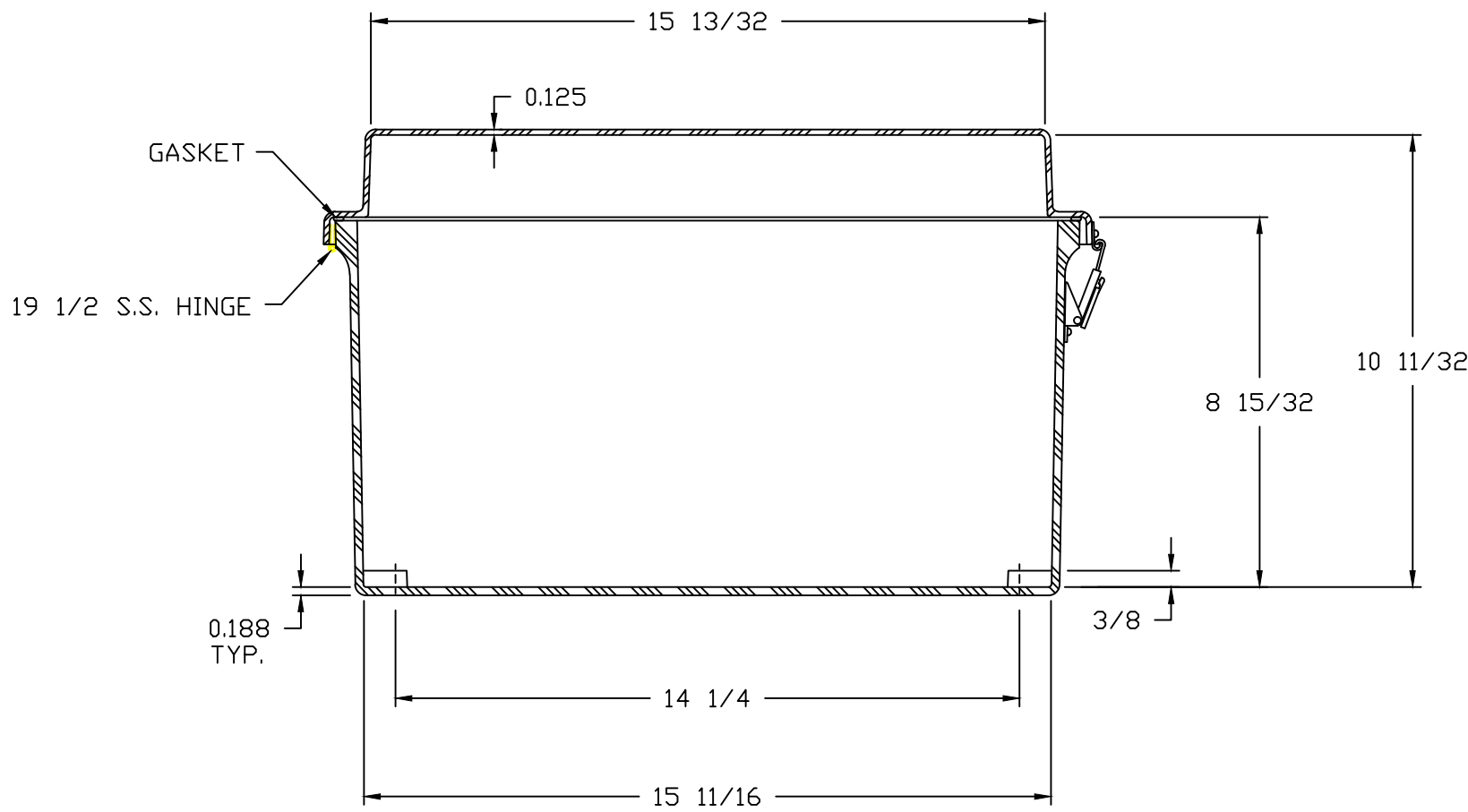
SECTION A-A
