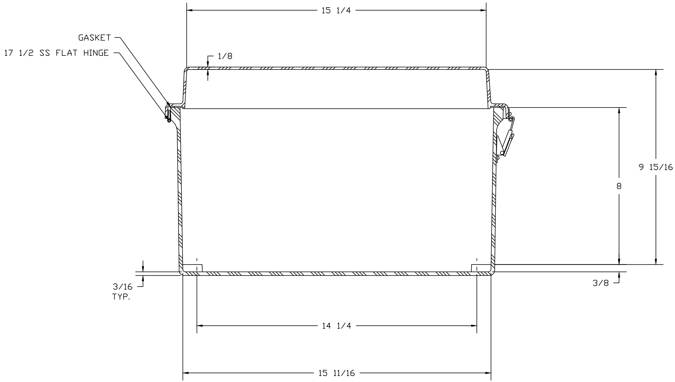
SECTION A-A
