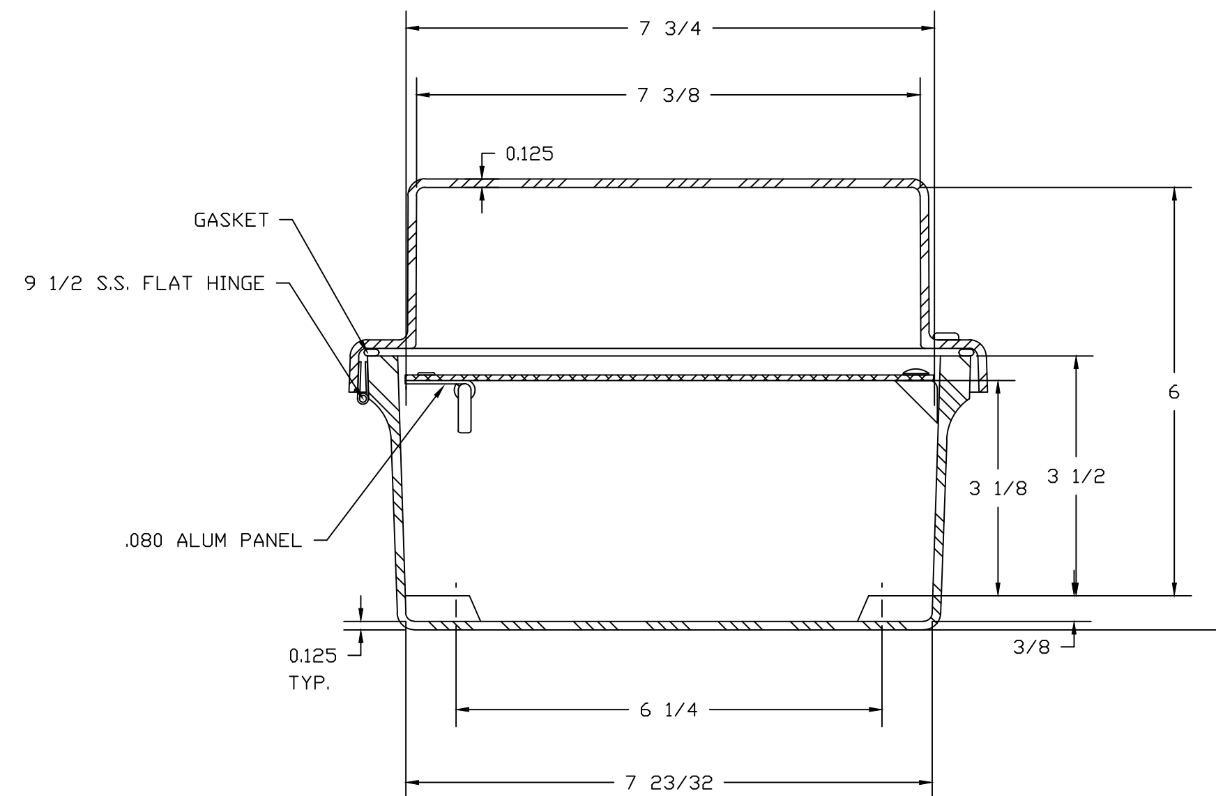
SECTION A-A
