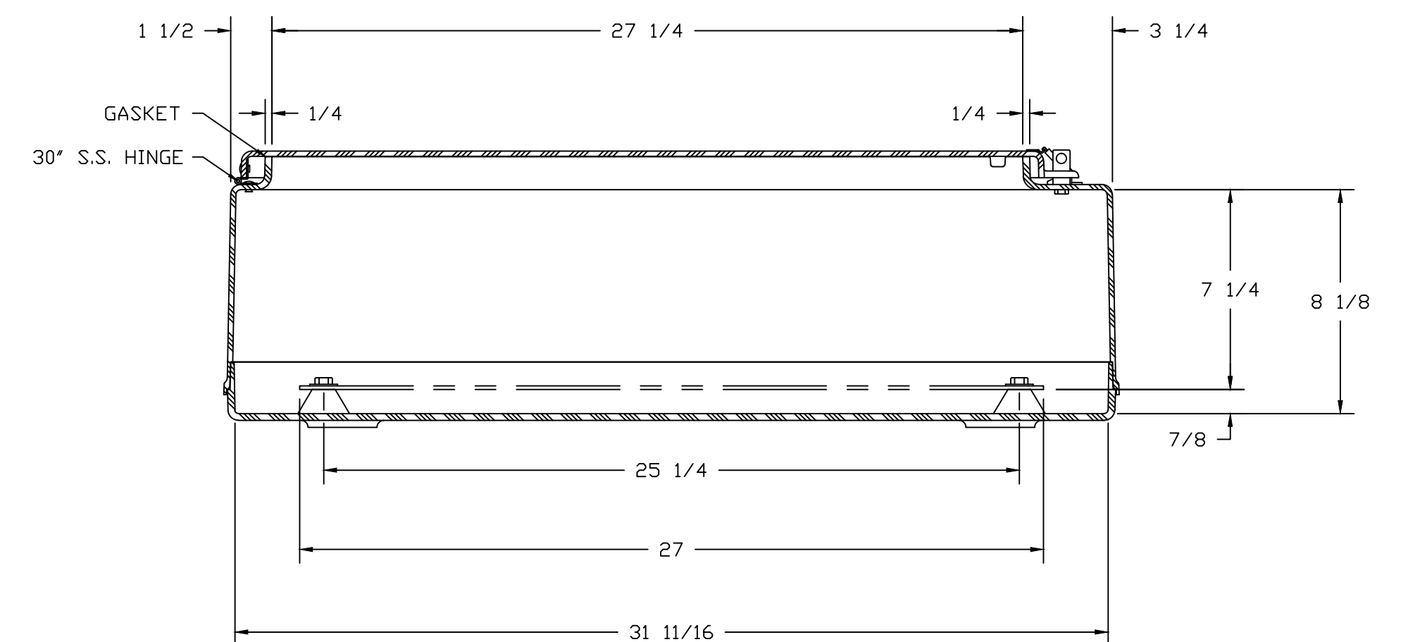
SECTION A-A
