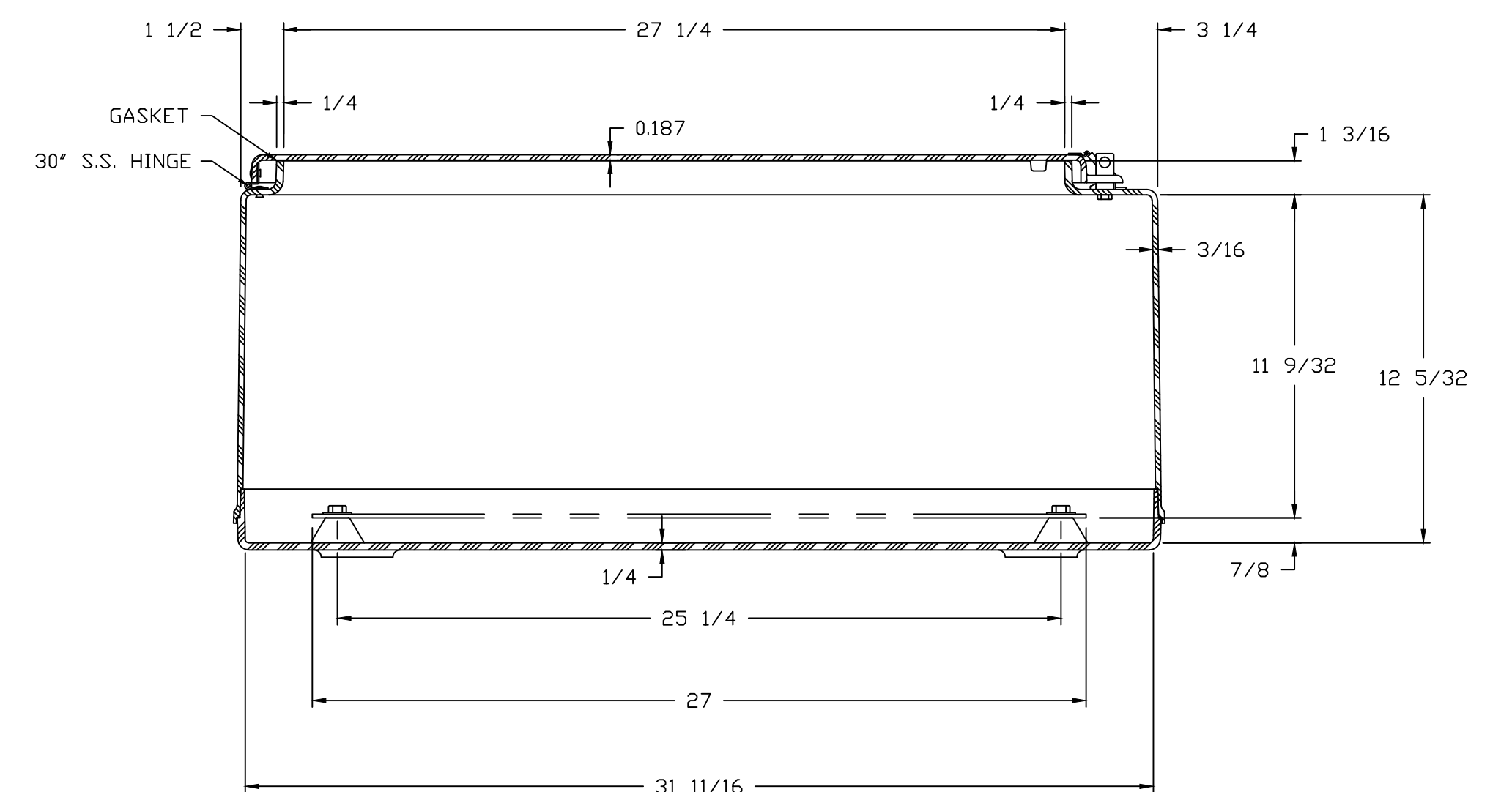
SECTION A-A
