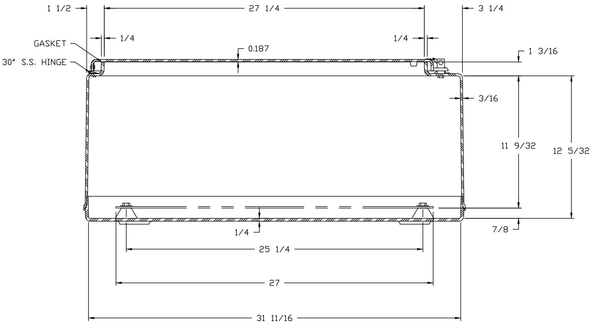
SECTION A-A
