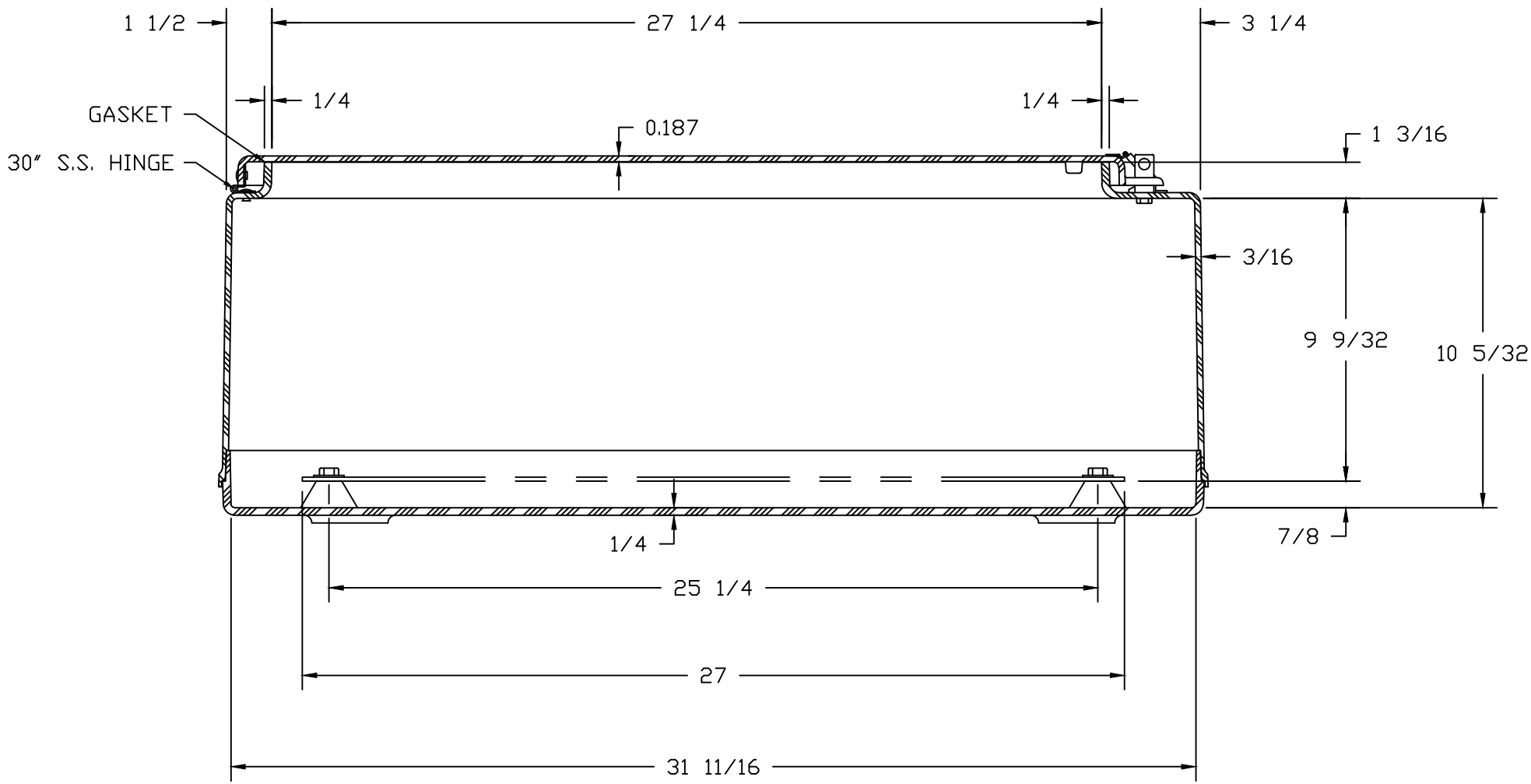
SECTION A-A
