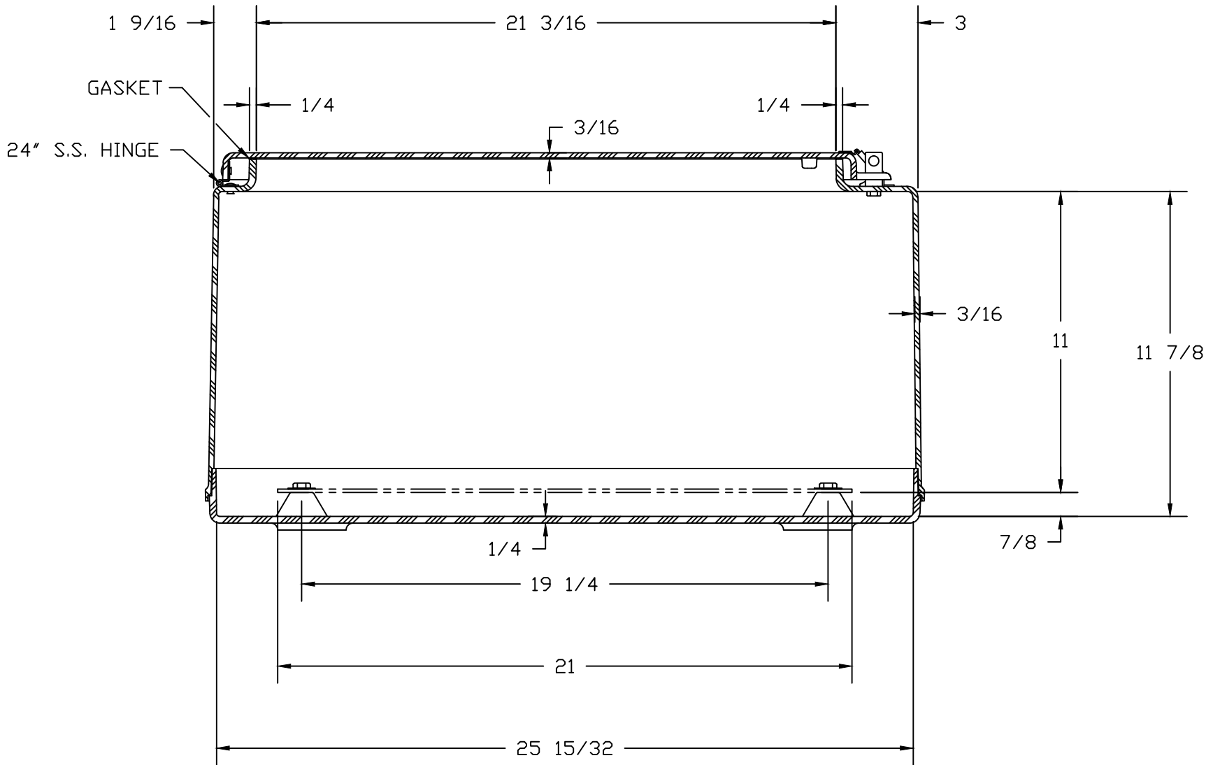
SECTION A-A
