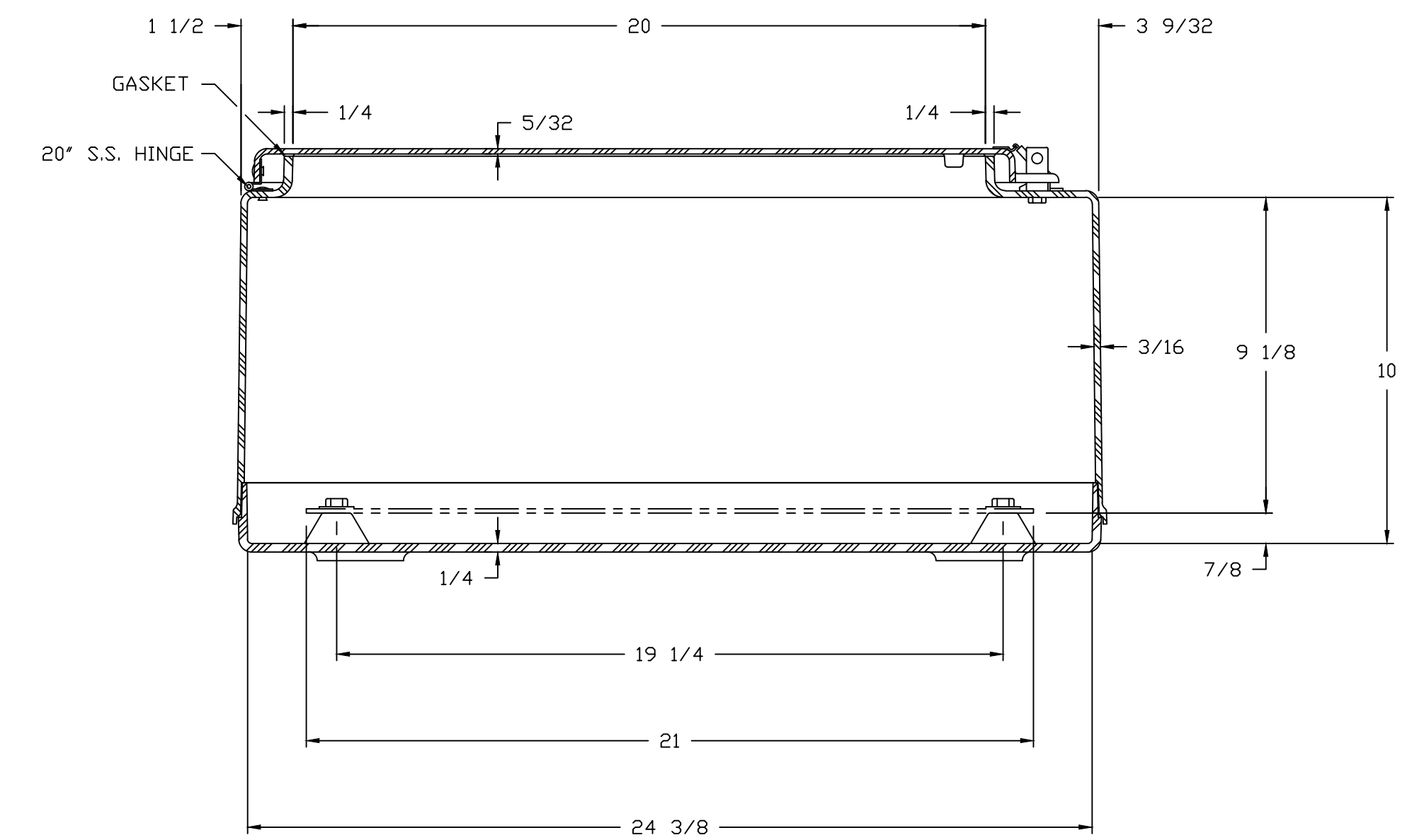
SECTION A-A
