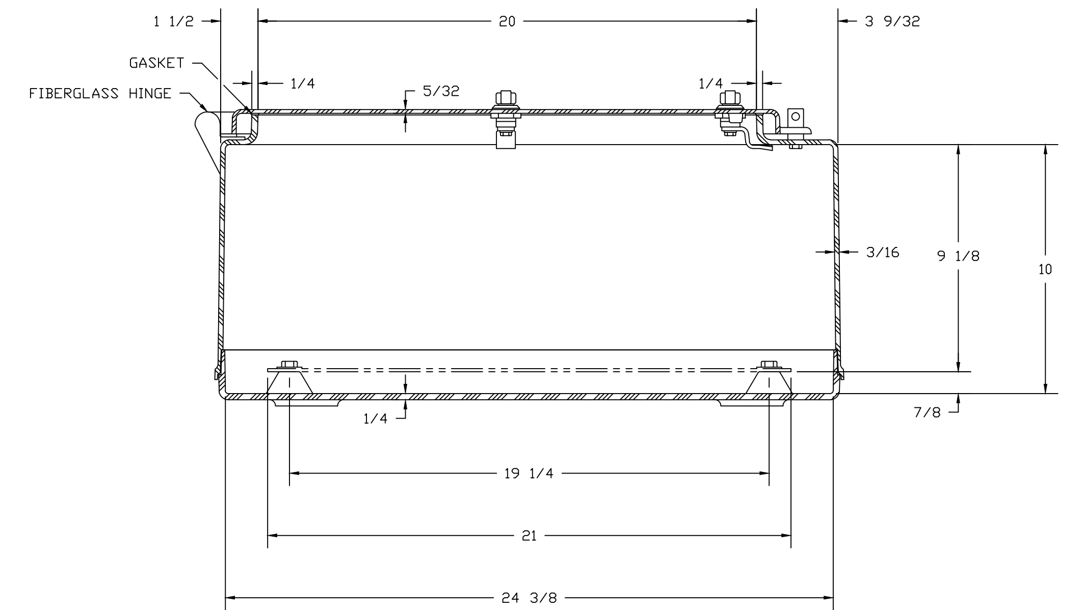
SECTION A-A
