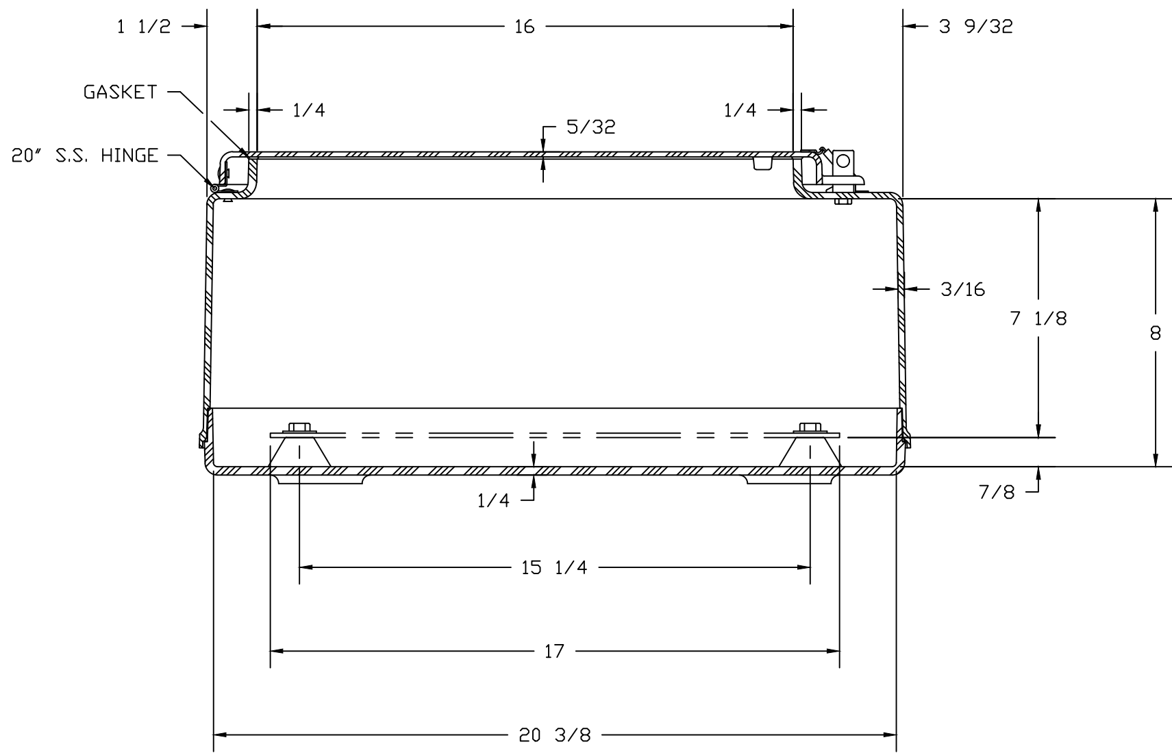
SECTION A-A
