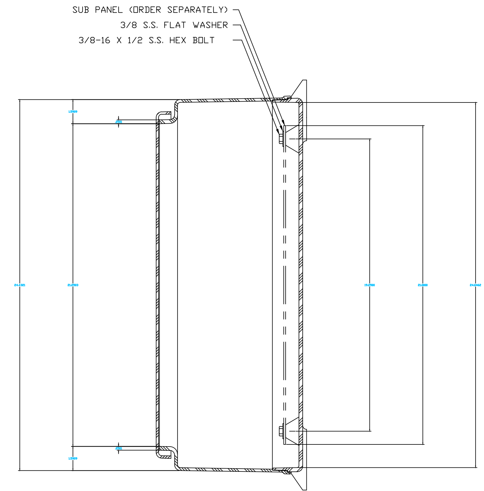
SECTION B-E
