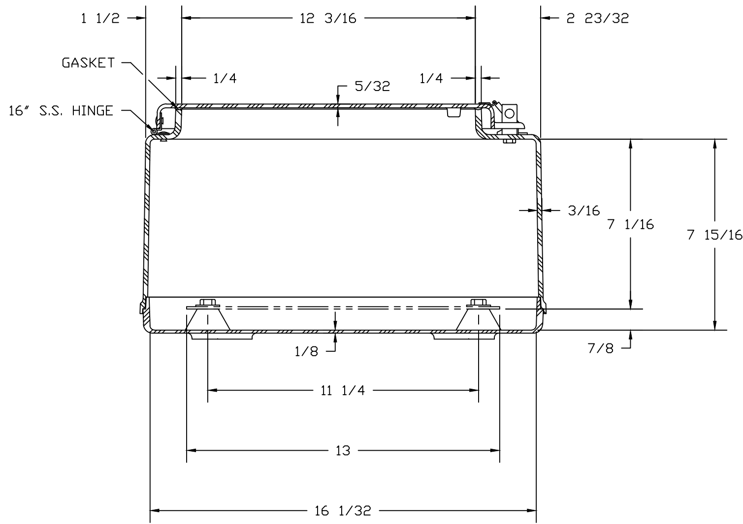
SECTION A-A
