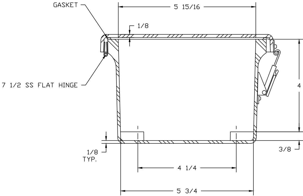
SECTION A-A
