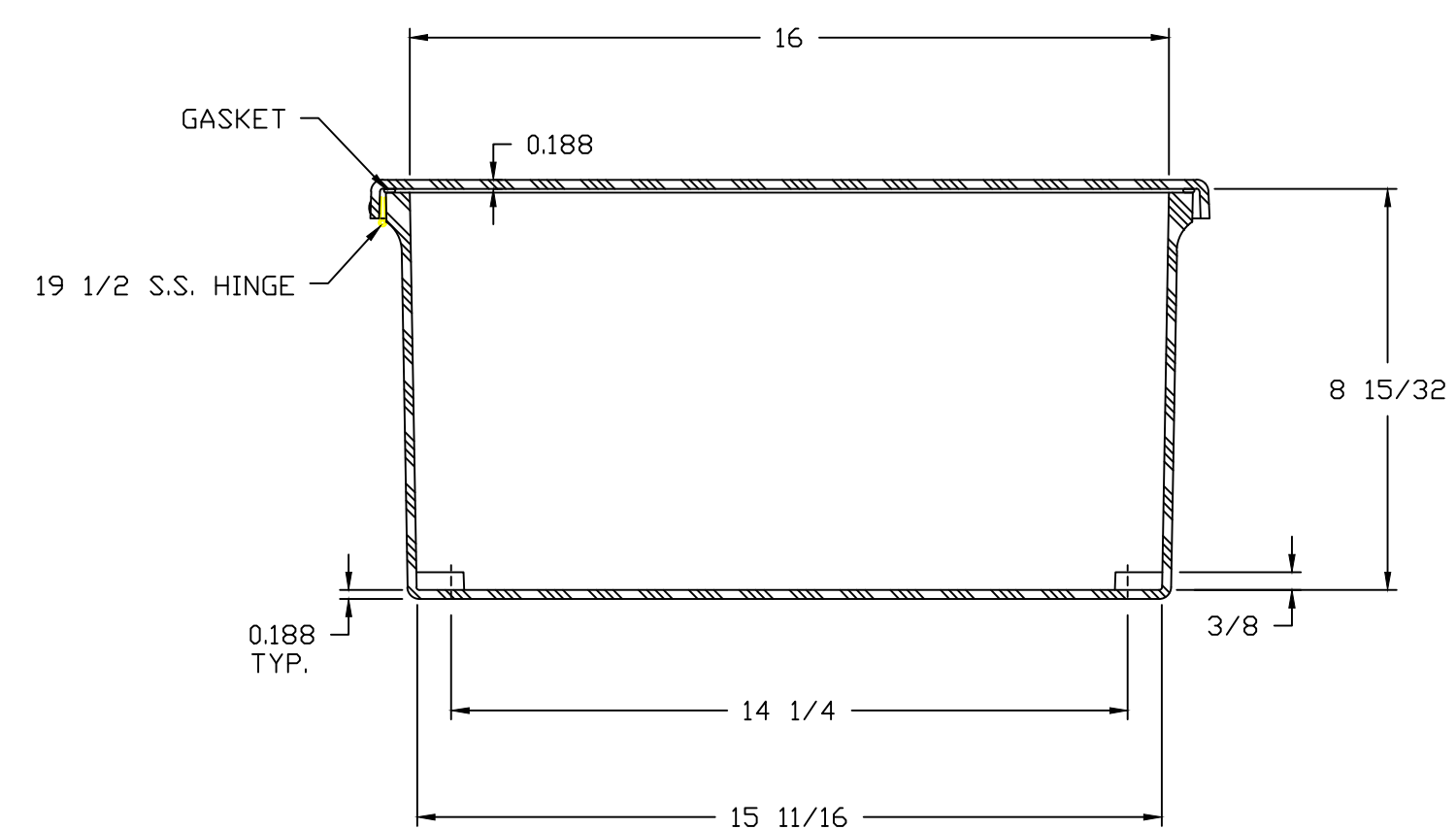
SECTION A-A
