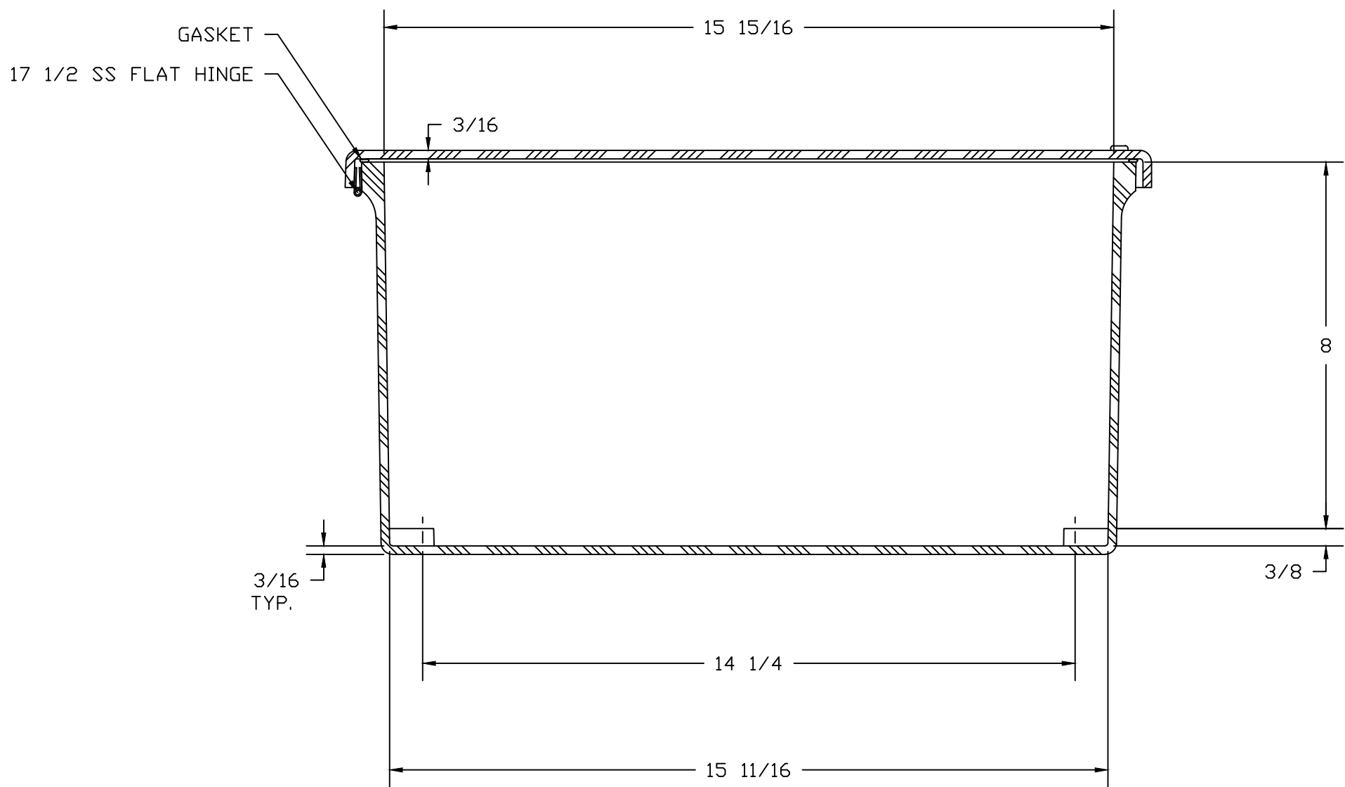
SECTION A-A
