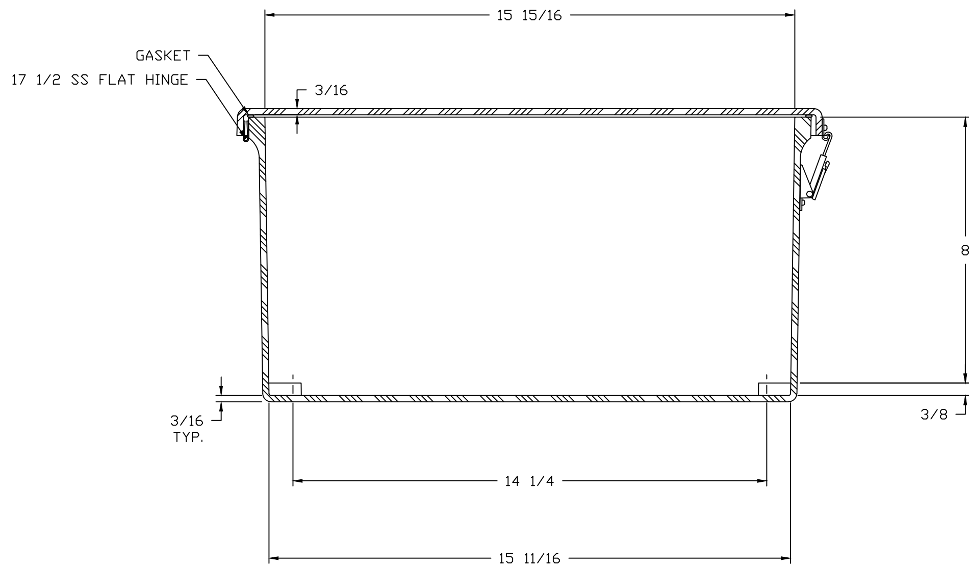
SECTION A-A
