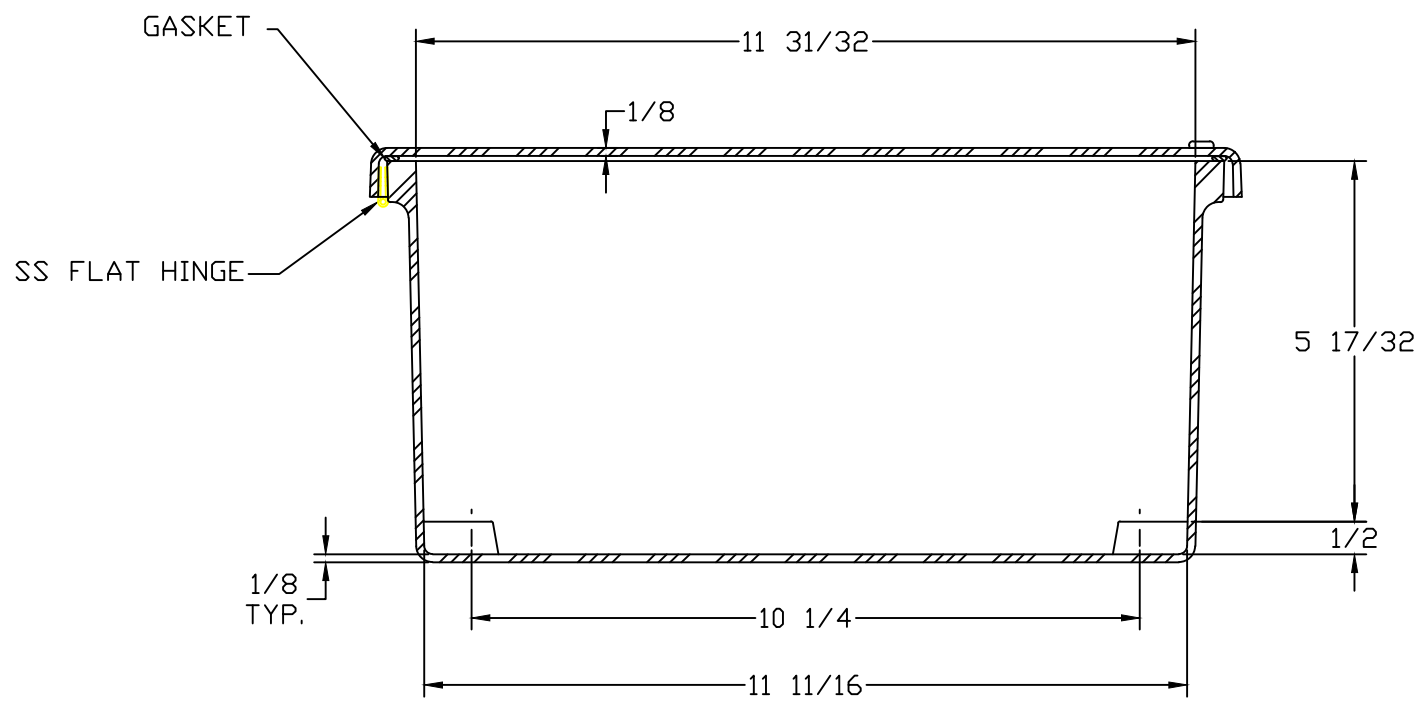
SECTION A-A
