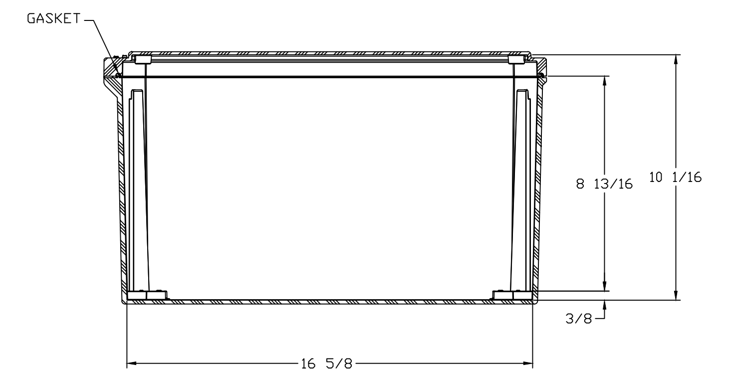
SECTION A-A
