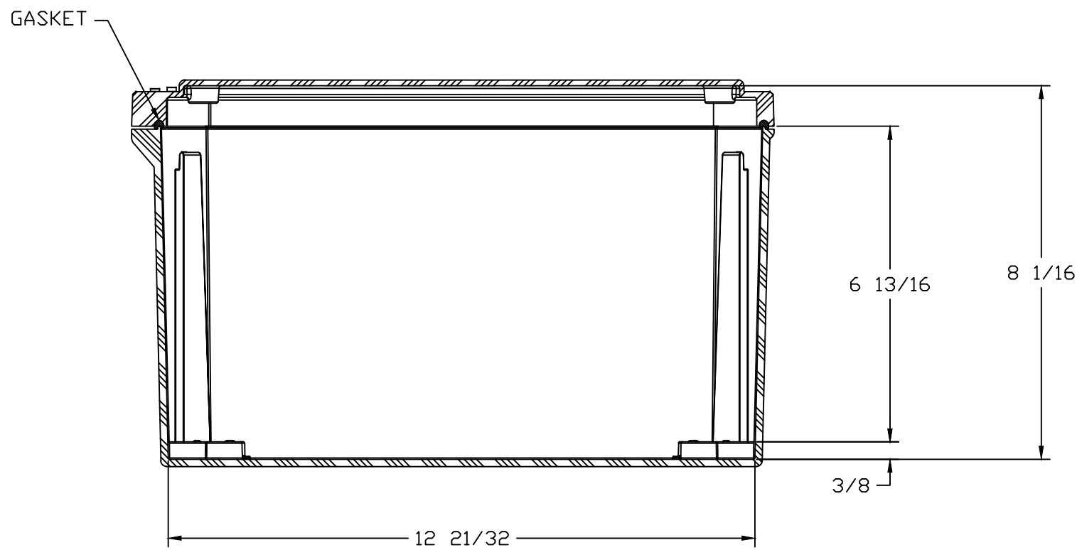
SECTION A-A
