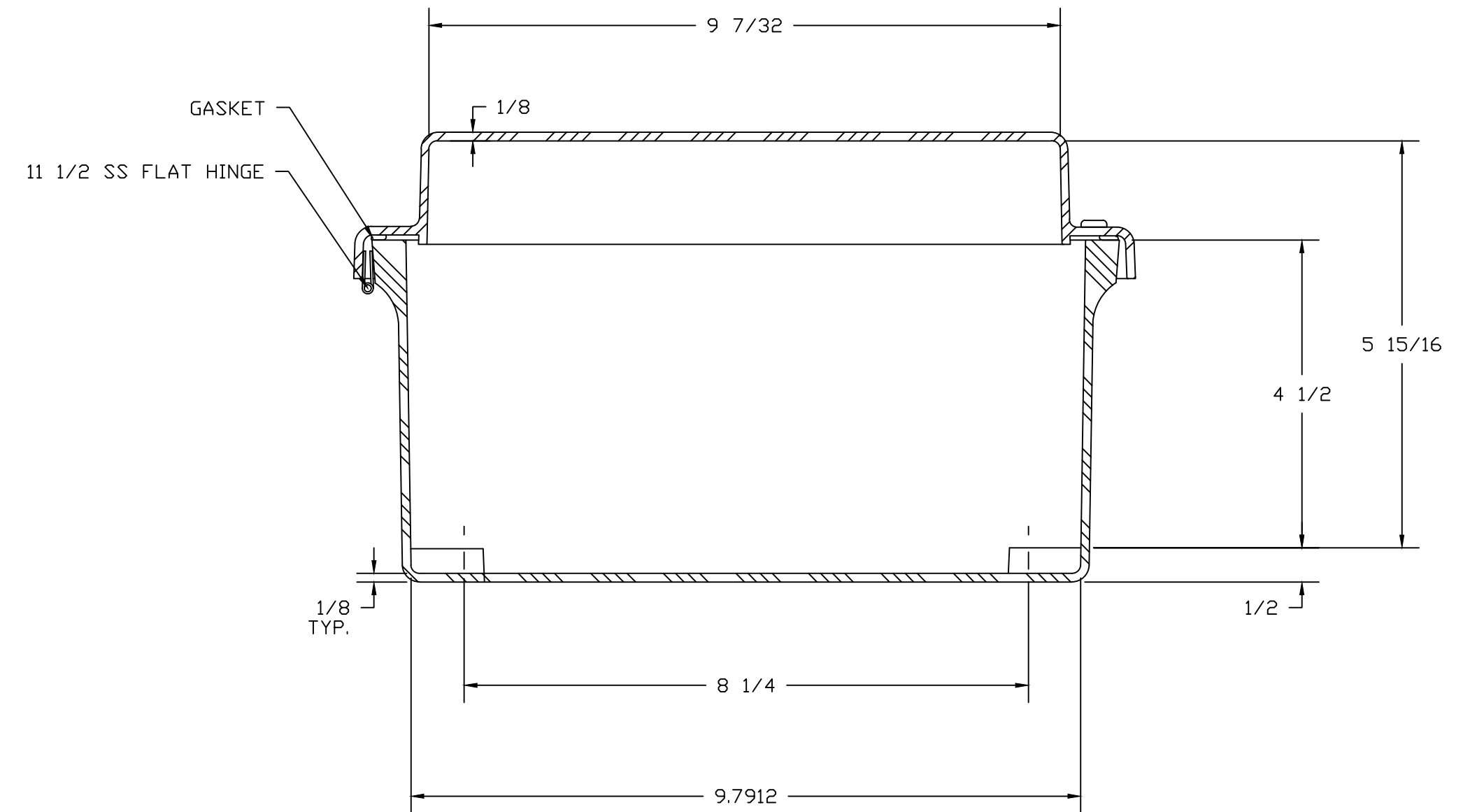
SECTION A-A
