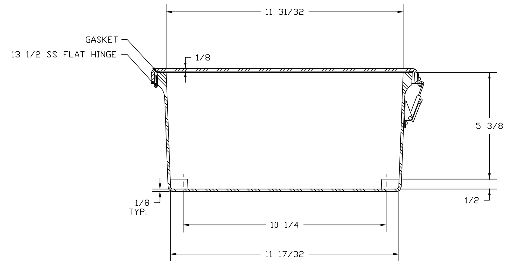
SECTION A-A
