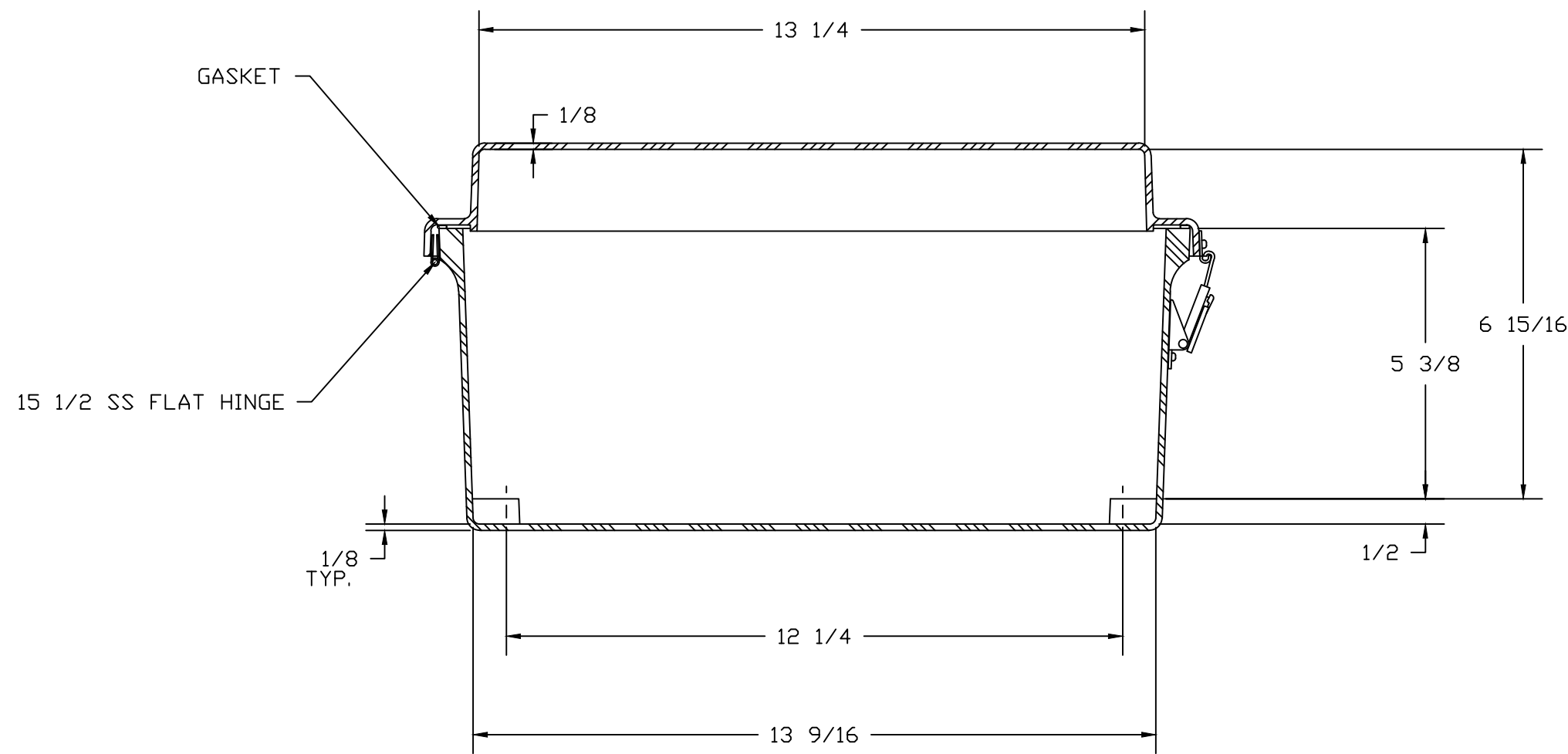
SECTION A-A
