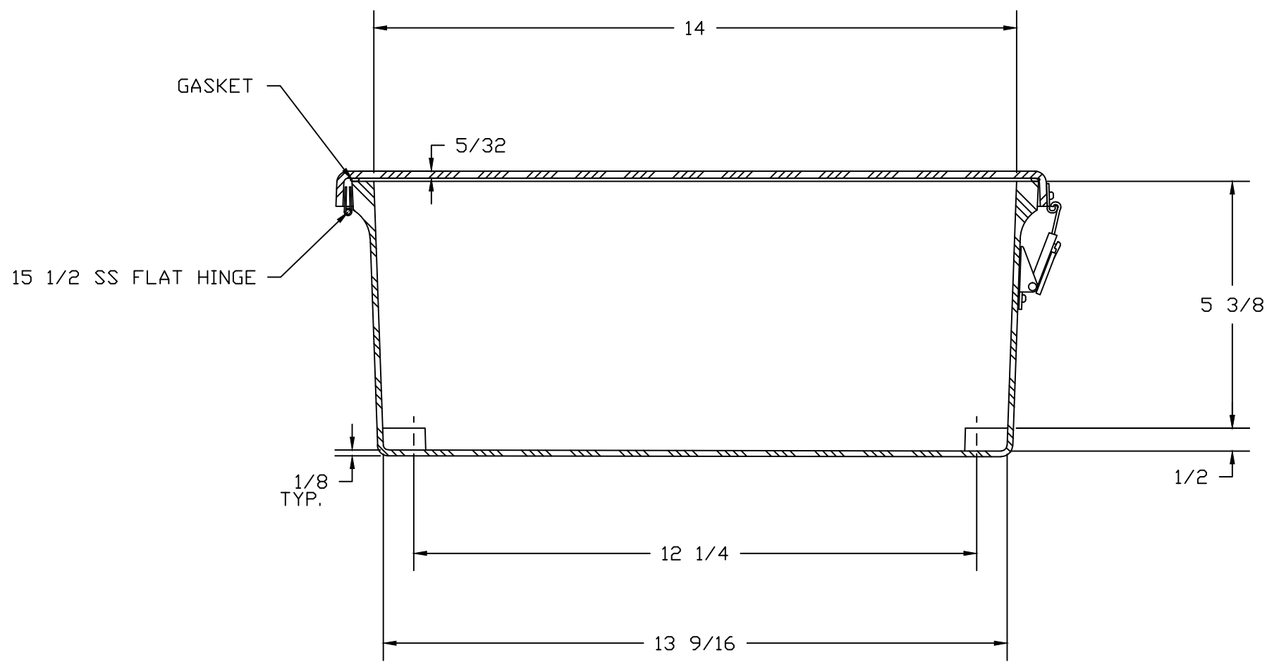
SECTION A-A
