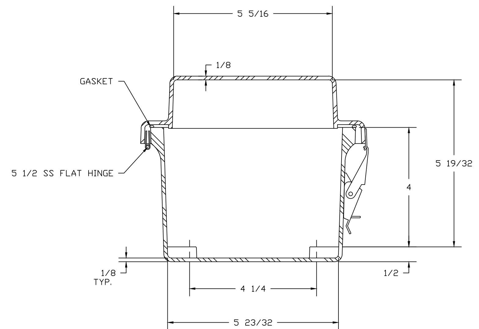
SECTION A-A
