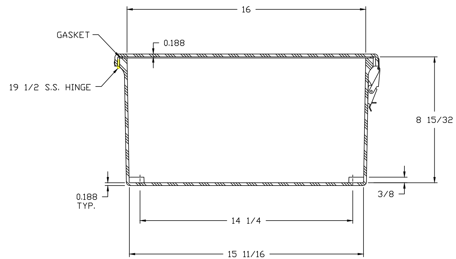
SECTION A-A
