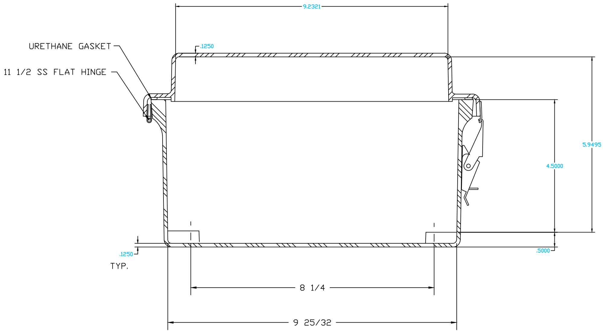
SECTION A-A
