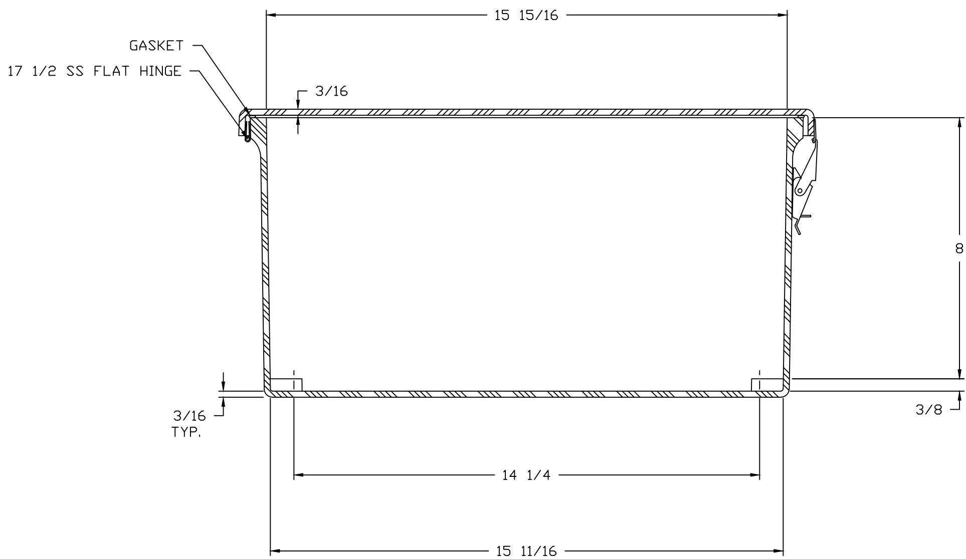
SECTION A-A
