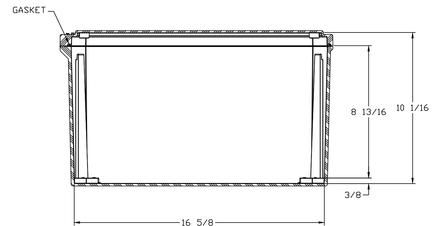
SECTION A-A
