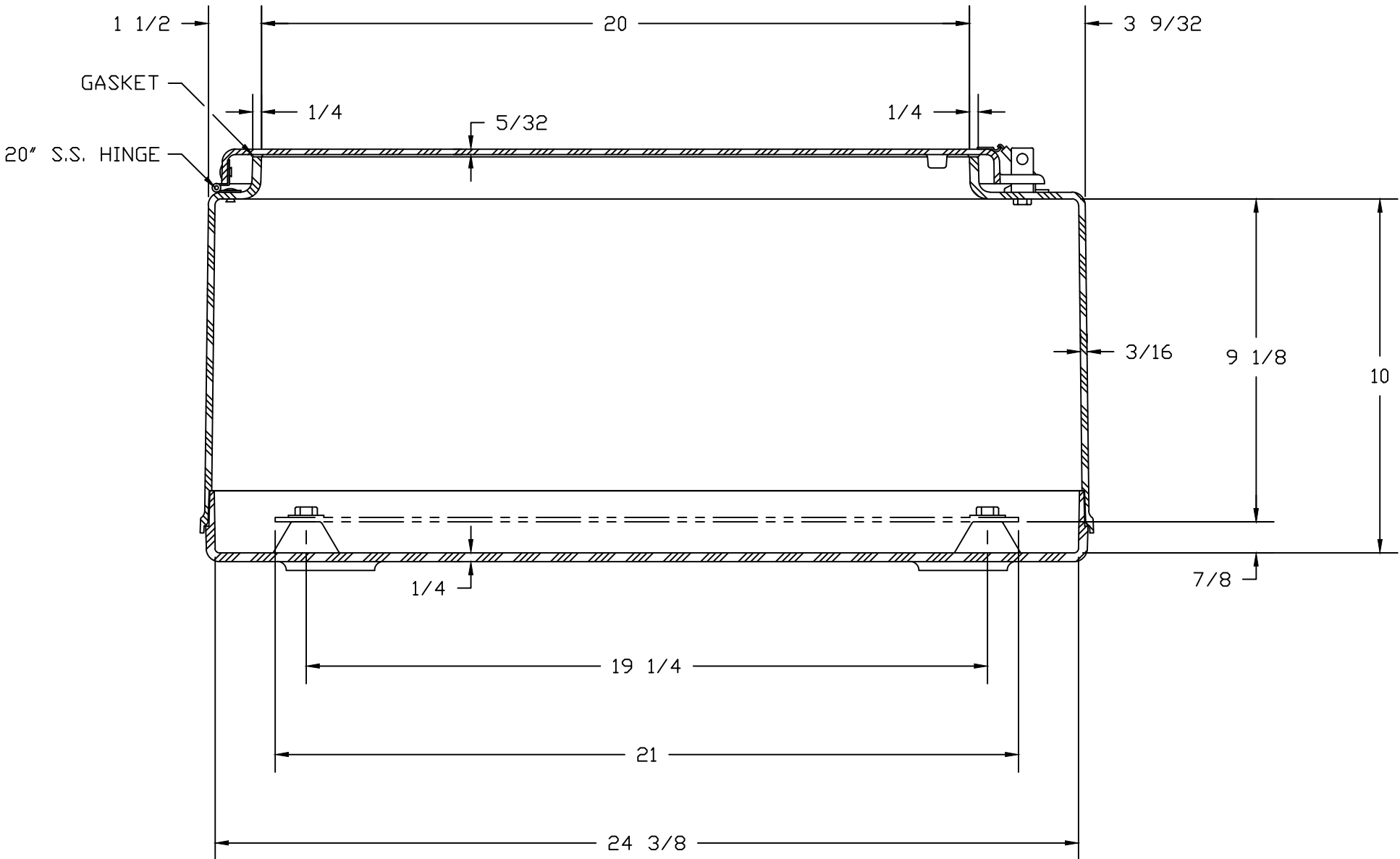
SECTION A-A
