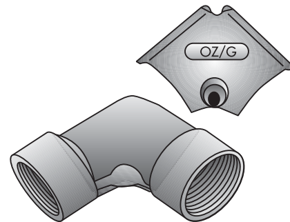
Type CE
