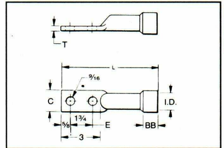
Type KC22B2 1/2-13 stud size
